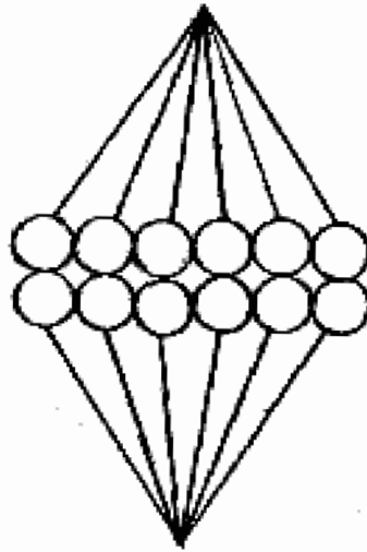
NEUTRINO
